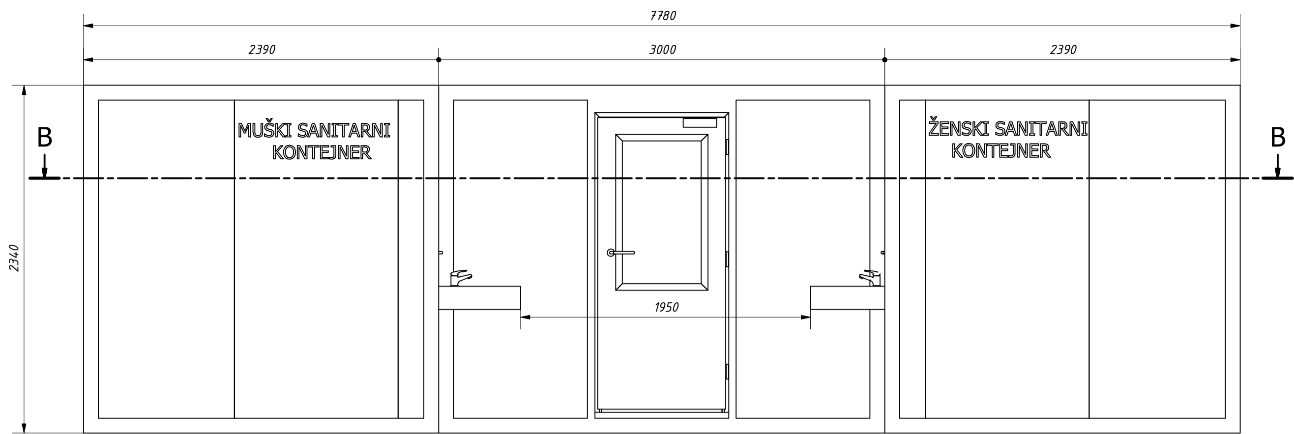
B-B ( 1 : 25 )
